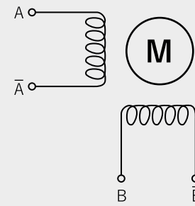
(図2・バイポーラ方式 Figure 2・Bipolar)
