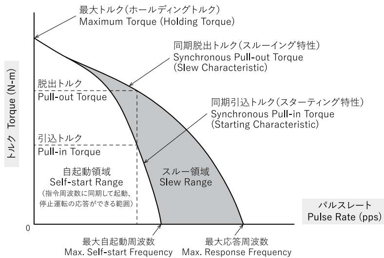
ステッピングモータ特性曲線 Torque Characteristics
