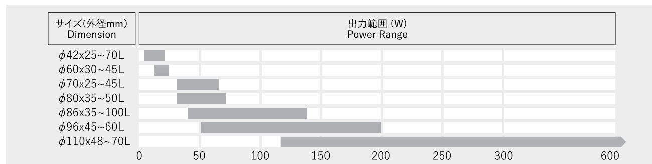
モータサイズ-出力相関表 (100V, 4P 連続~短時間) Size and Output Power
