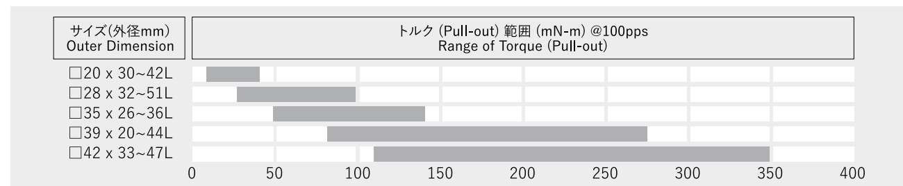
モータサイズ・トルク(Pull-out)相関表 Size and Torque (Pull-out)
