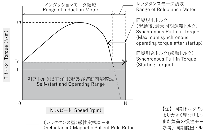
ACシンクロナスモータ特性曲線 Torque Characteristics of AC Synchronous Motor
